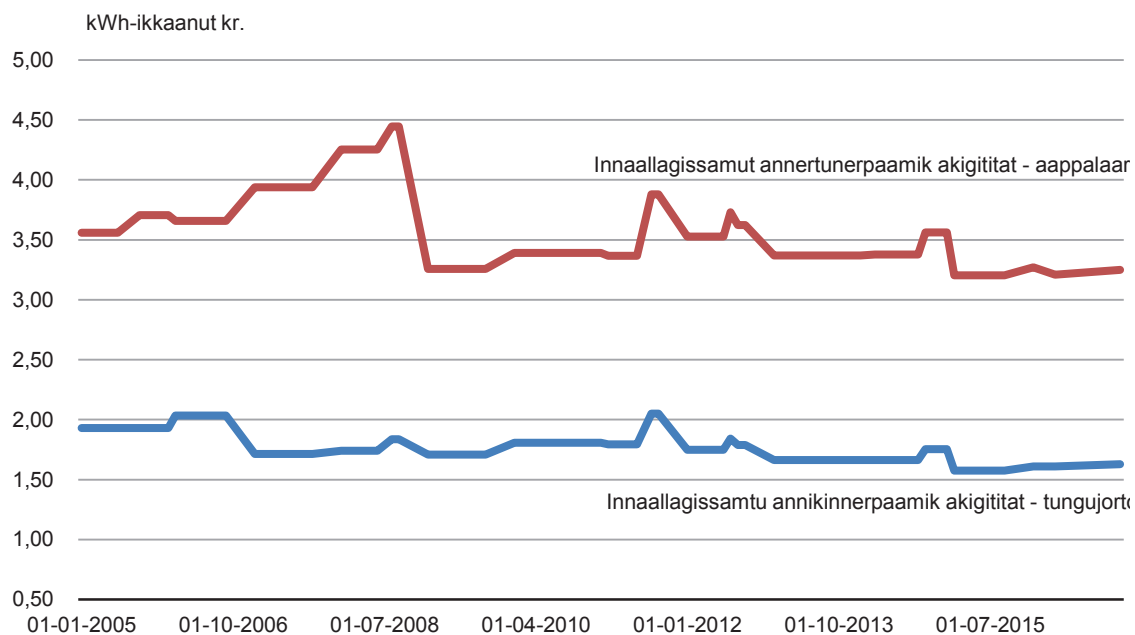
Ilusiliaq 1 2004-2017-imi innaallagissamut akiusuni agguaqatigiissitatut allanngoriartorerit (akit 2016-imeersut) Najoqutaq: Nukissiorfiit
