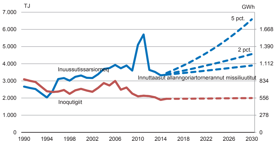
Ilusiliaq 16. 1990-2015-imut inaarutaasumik nukissiuuteqarnermik atuineq, 2016-2030-mut siumut inissiineramik ilanngussivigalugu
