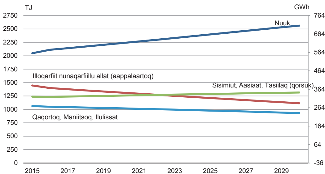
Ilusiliaq 17. Illoqarfinnut nunaqarfinnullu agguataarlugit innaallagissamut kiassarnermullu nukissiuuteqarnermik atuinermik siumut inissiineq, 2015-2030. Saamiata aamma talerpiata tungaanni titarnerit napasut nukissiuuteqarnermik atuineq Terajoule'tut aamma Gigawatt'itut nal. akunnerinut takutitsipput.
