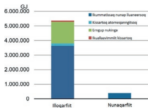
Ilusiliaq 11. 2015-imi illoqarfinni aamma nunaqarfinni innaallagissamut kiassarnermullu nukissiuuteqarnermik atuineq ataatsimoorussaq (GJ)
