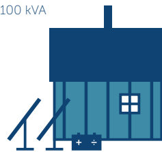
IKERASAARSUK Seqernup qinggorneranik katersiviit Panelit 240/78 kWp Batteriillu 167 Kwh/100 kVA
